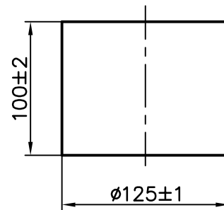
1x Verbindingsstuk D125
