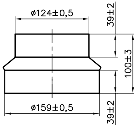
2x Verloopstuk D160 – D125
