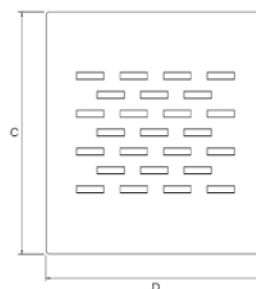
alpha-Luftdurchlass DN 125
