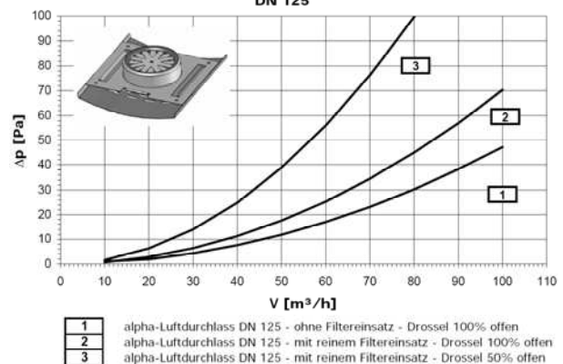
alpha-Luftdurchlass DN 125
